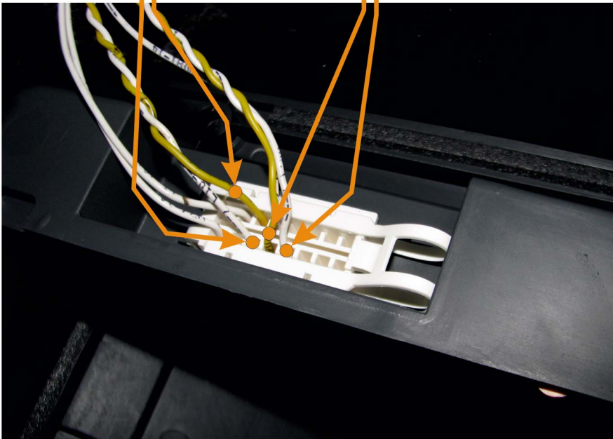
Разъём за сиденьем водителя
