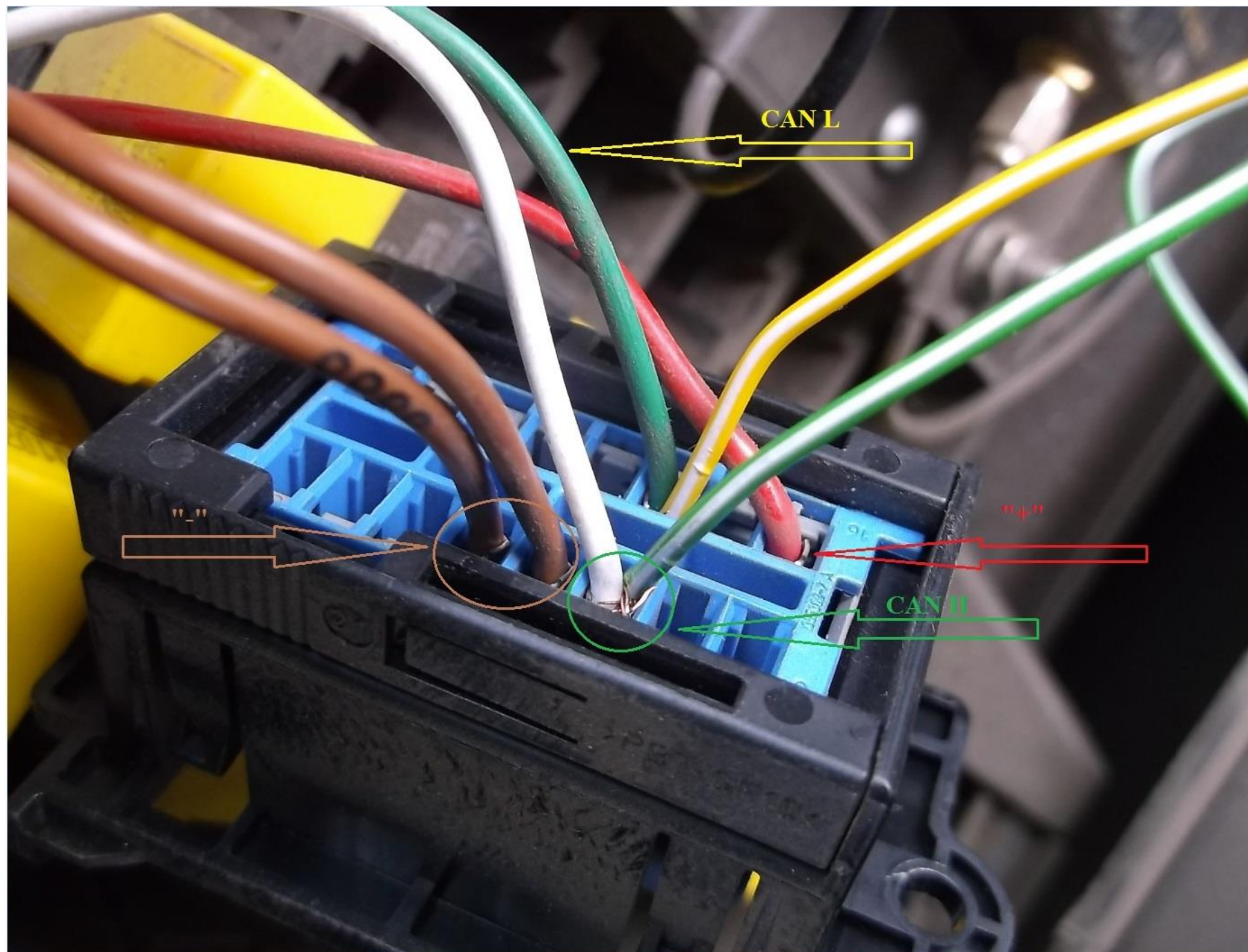
Разъём OBD-2
