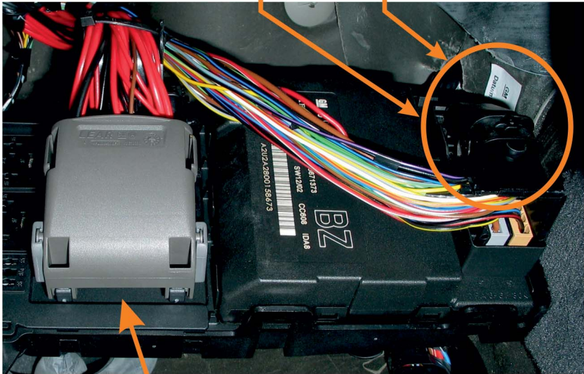
УПРАВЛЯЮЩИЙ МОДУЛЬ
