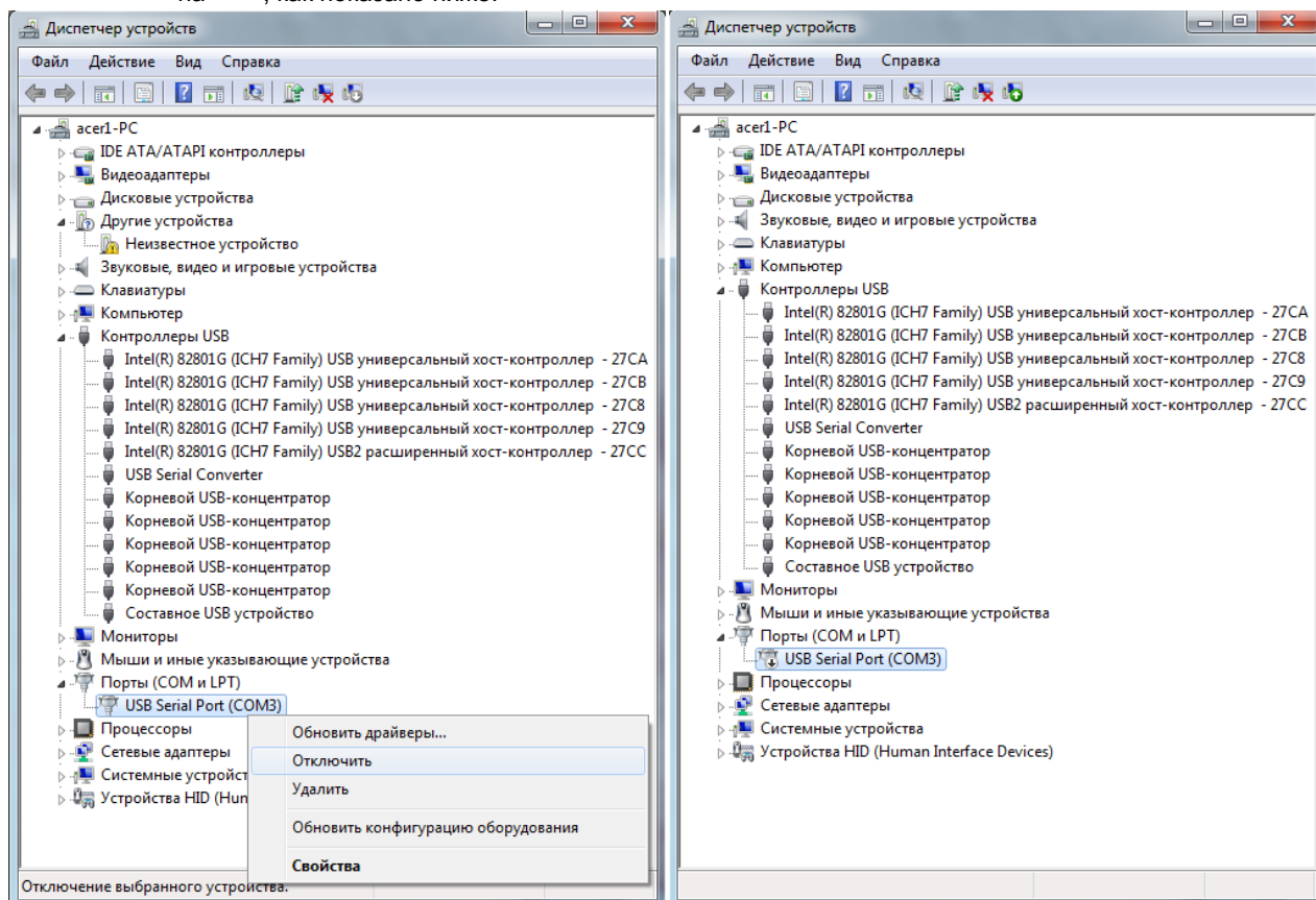
Рис.41 – Установка драйверов для Microsoft Windows 7.
