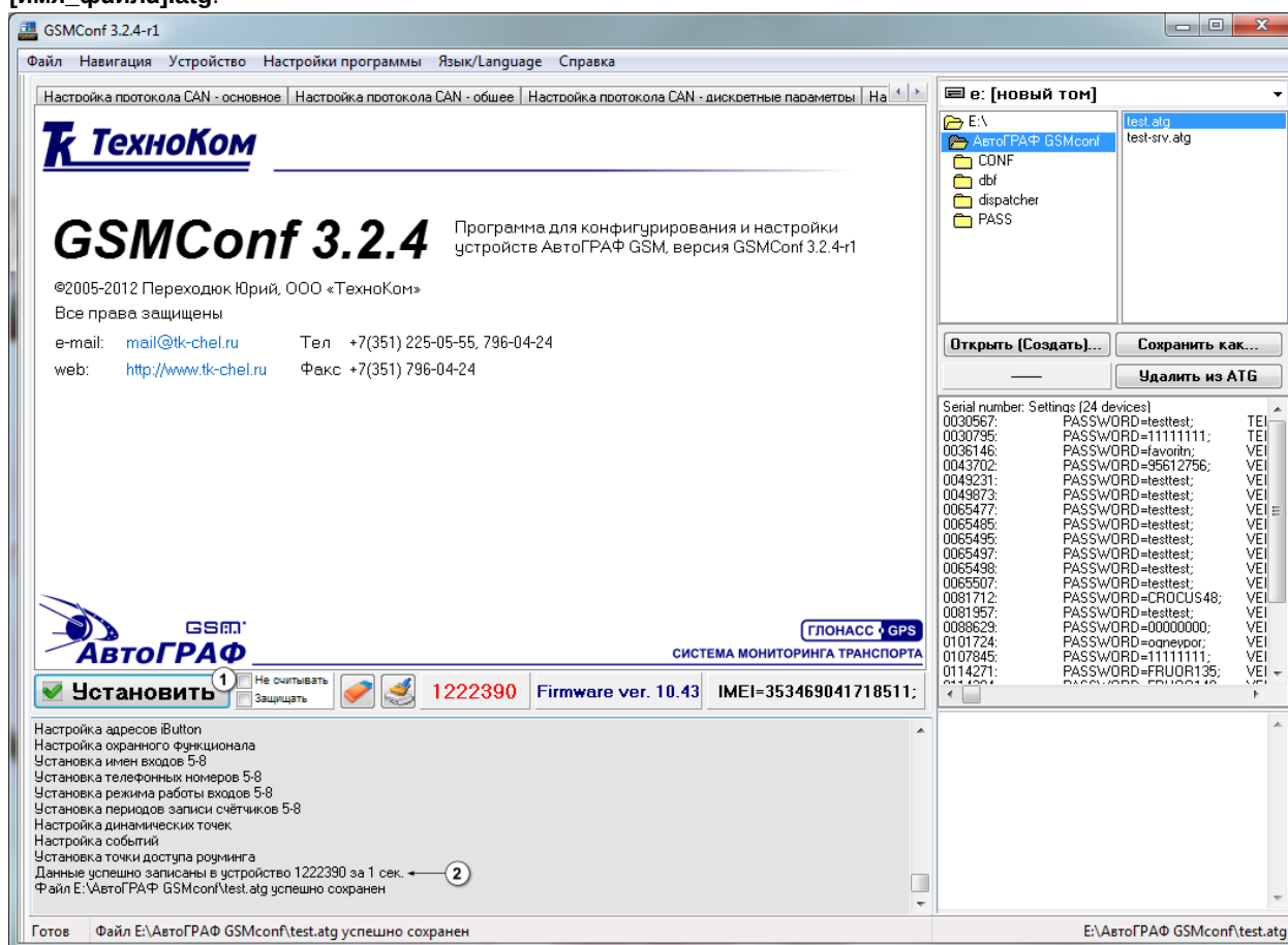
Рис.40 – Запись настроек в терминал.
