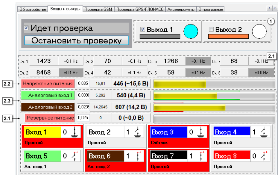
Рис.45 – Вкладка «Контроль. Входы и выходы».
