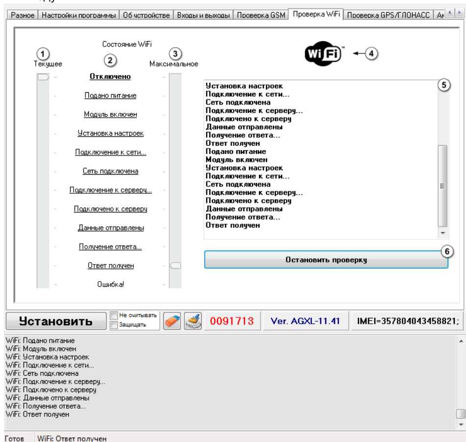
Рис.53 – Вкладка Контроль. Проверка WiFi.
