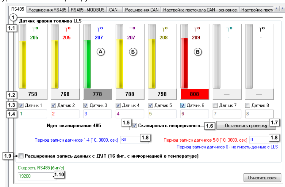
Рис.27 – RS-485.
